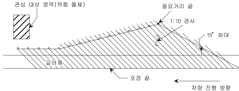
<그림 2.21> 차도에서 방호울타리까지의 경사와 퍼짐률
