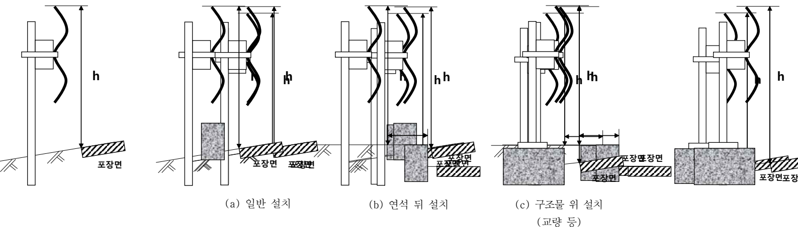
〈그림 2.17〉 방호울타리 높이 측정 예
