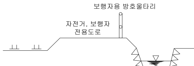
⑥ 자전거, 보행자 전용 도로 등에서의 방호울타리의 설치 예
