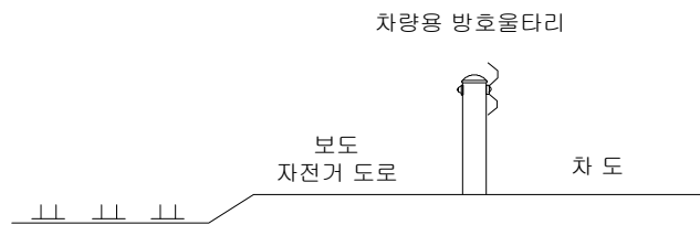
③ 차량 방호 보도용 방호울타리를 설치한 예(길 밖이 위험하지 않은 경우)
