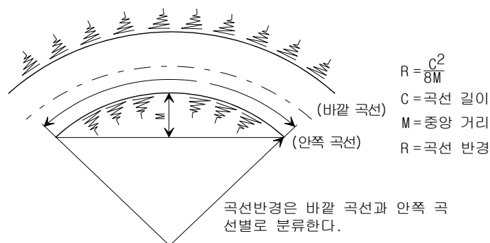
〈그림 2.26〉 곡선 구간의 곡선 반경 산출 방법
